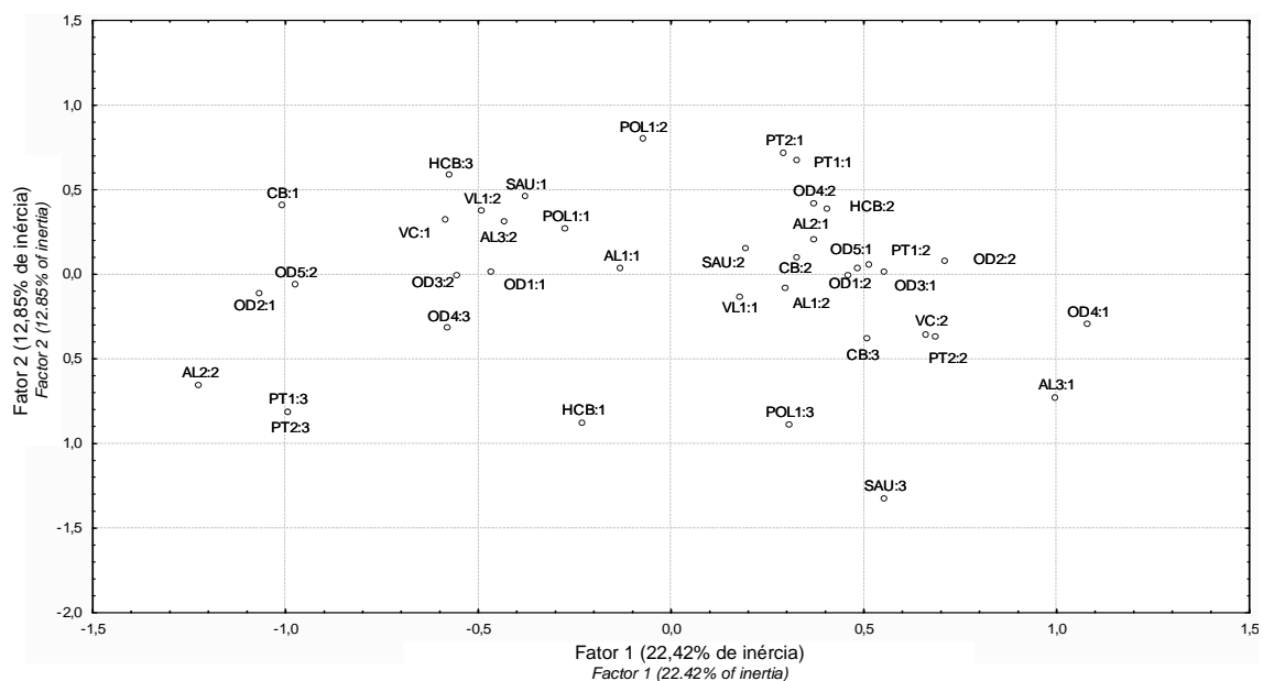
Figura 2. Gráfico mostra as variáveis/modalidades no plano fatorial F1 x F2.
