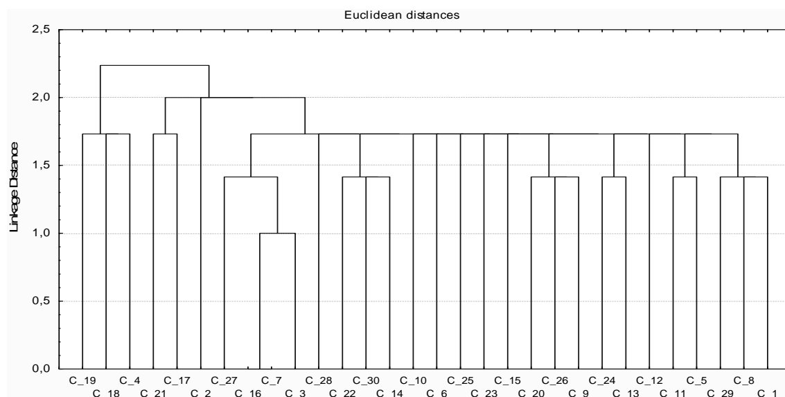
Figura 4. Dendrograma da análise de classificação hierárquica ascendente para um grupo de 30 agricultores da Área de Desenvolvimento Integrado de Colorado – Estado do Paraná.
