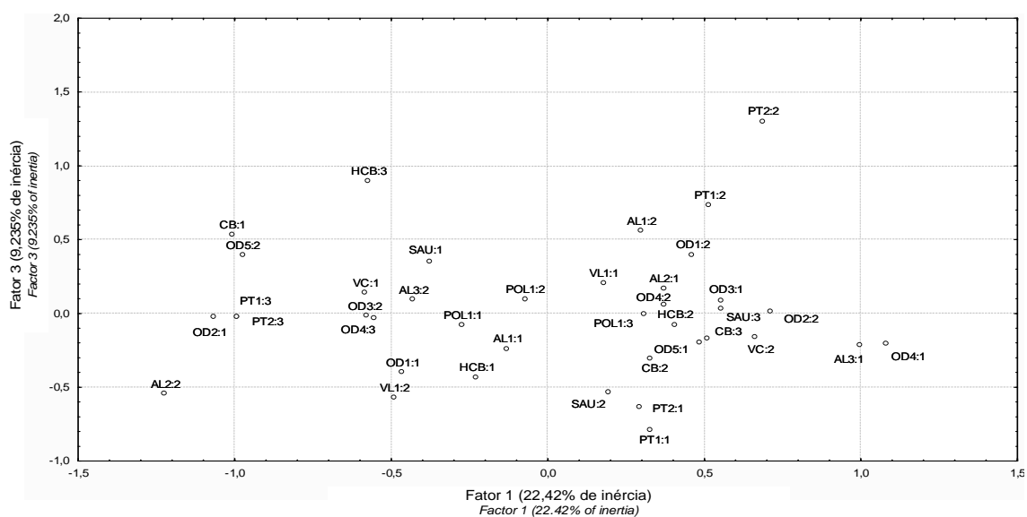
Figura 3. Gráfico mostra as variáveis/modalidades no plano fatorial F1 x F3.
