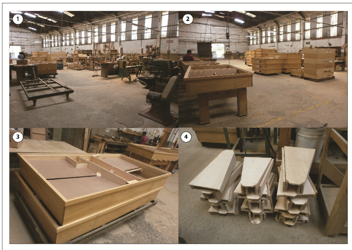
Figura 20: Visão parcial do Setor de montagem final das mesas para bilhar. Em destaque na foto 1 alguns equipamentos e máquinas, principalmente a esteira onde são colocadas as mesas em processo de produção para o deslocamento pela fábrica; na foto 2 algumas mesas em fase final de montagem; na foto 3 duas mesas ainda sem os pés e tampos, verifica-se o mecanismo de rolamento das bolas no interior da mesa. Na foto 4 peças que irão compor o interior da mesa.
