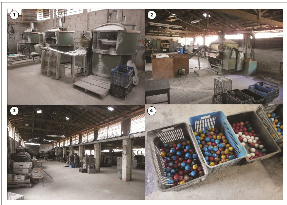
Figura 27: Setor de fabricação de equipamentos e máquinas adaptadas / Finalização das bolas. Neste setor encontram-se máquinas como a lixadeira (foto 1) e a polidora (foto 2) de bolas. Por meio da foto 3 tem-se uma na visão parcial deste setor. Nesta área foram criadas/adaptadas as máquinas e equipamentos utilizados por Antonio Hernandez junto aos seus empregados e colaboradores. O produto acabado (bola) pode ser visualizado na foto 4
