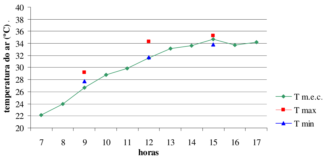
Gráfico 5.42 – Comparação entre a temperatura do ar (°C) na praça e na mini-estação climatológica – P2 – Verão
