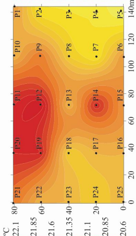
Figura 5.26 - P1 - Inverno/ 9h00min/ distribuição da temperatura no piso (°C)
