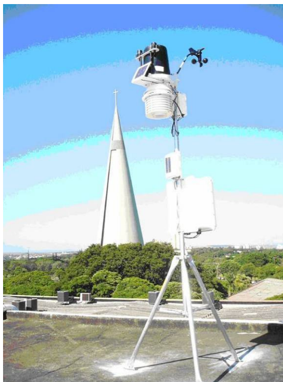
Figura 4.4 – Mini-estação climatológica
