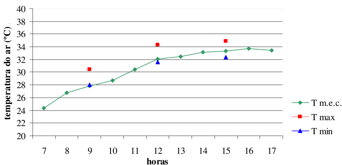
Gráfico 5.38 – Comparação entre a temperatura do ar (°C) na praça e na mini-estação climatológica – P1 – Verão
