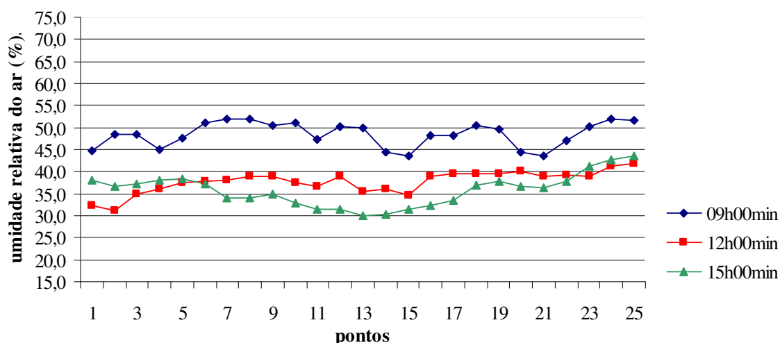
Gráfico 5.7 – Variação da umidade relativa do ar (%) por pontos e horário - P1 – Outono
