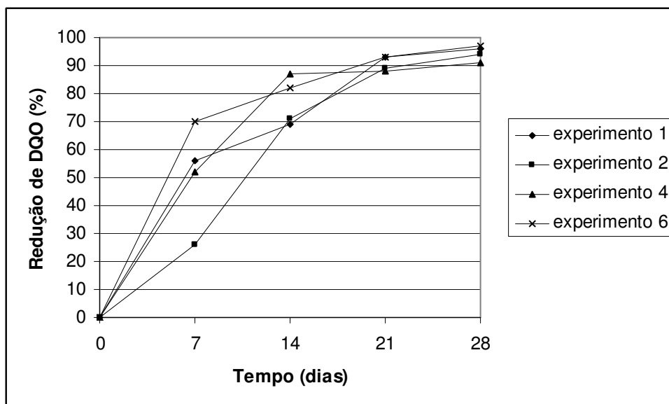
Figura 16 Redução média de DQO solúvel nos experimento 1, 2, 4, e 6 ao longo do tempo de operação
