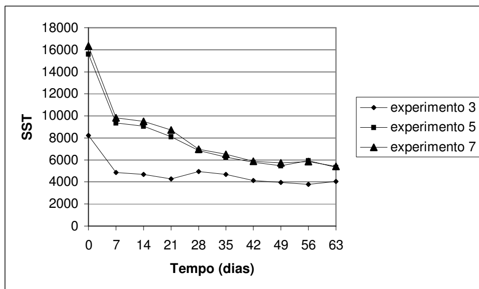
Figura 11 Avaliação média dos SST nos experimentos 3, 5 e 7 com tempo de operação de 60 dias
