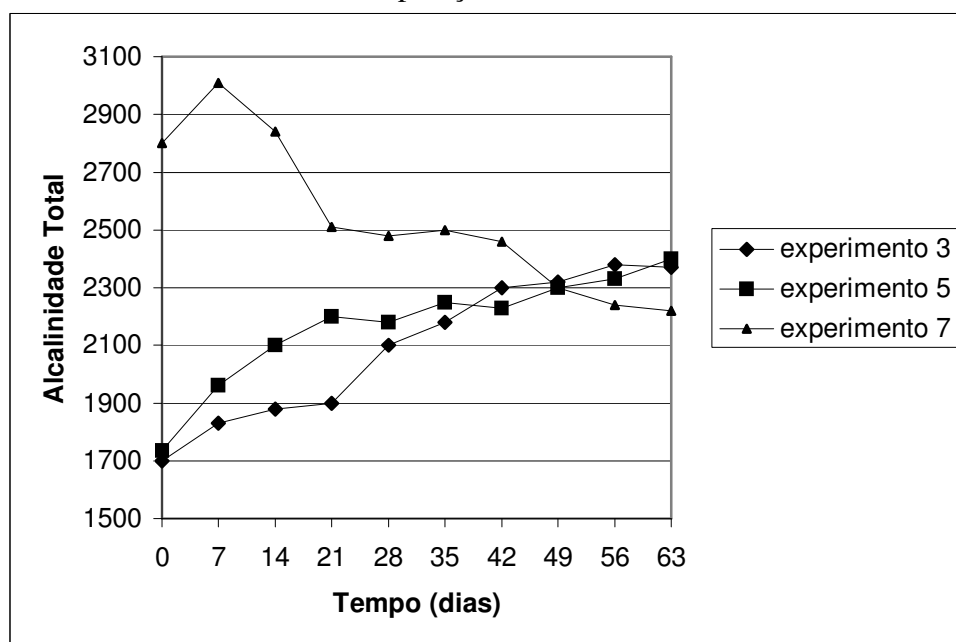
Figura 7 Avaliação média da alcalinidade total nos experimentos 3, 5 e 7 com tempo de operação de 60 dias
