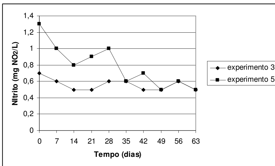
Figura 21 Evolução da concentração de nitrito no sobrenadante, nos experimentos 3 e 5 ao longo do tempo de operação
