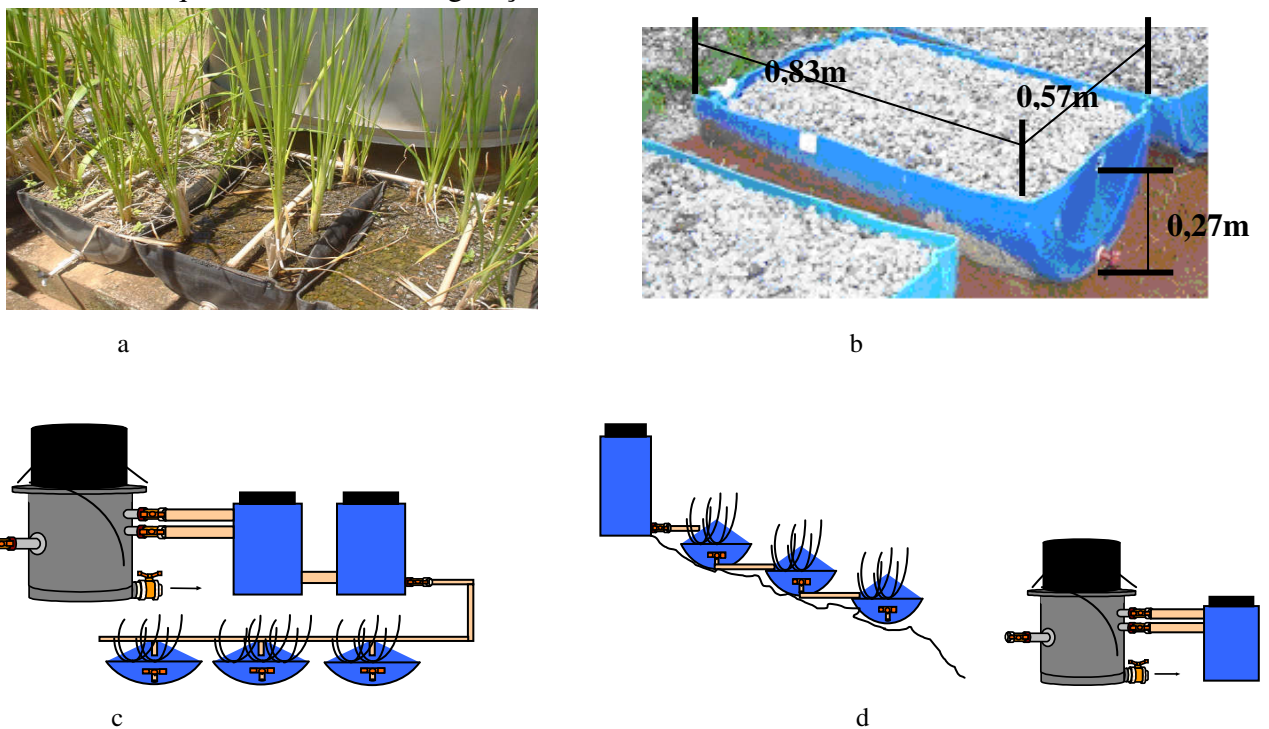
Figura 3.4 - (a) Leitos cultivados; (b) dimensões do leito; (c) configuração em paralelo; (d) configuração em série
