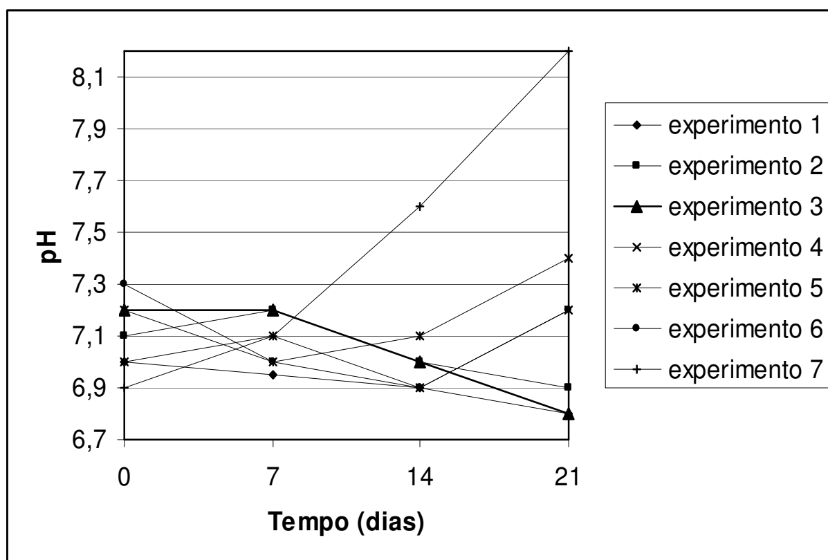
Figura 24 Resultado do pH dos leitos cultivados com Taboas nos experimentos
