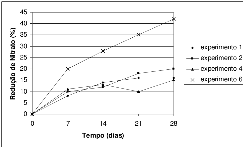
Figura 18 Redução média da concentração de nitrato no sobrenadante, nos experimentos 1, 2, 4, e 6 ao longo do tempo de operação
