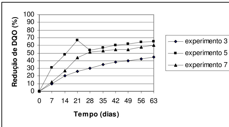
Figura 15 Redução média de DQO total nos experimento 3, 5 e 7 ao longo do tempo de operação
