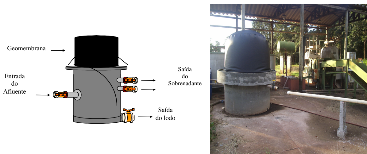
Figura 3.2 – Biodigestor de baixa carga
