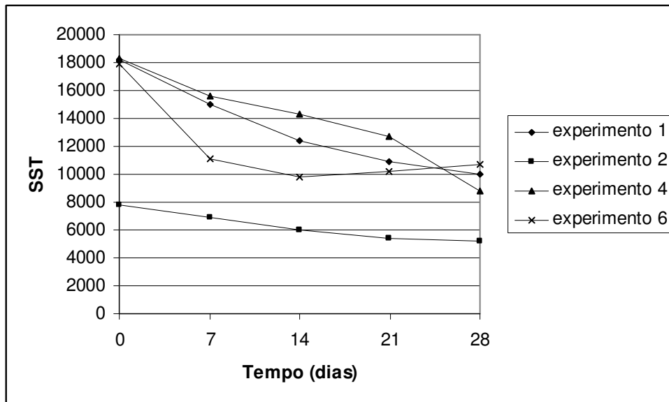
Figura 10 Avaliação média dos SST nos experimentos 1, 2, 4 e 6 com tempo de operação de 30 dias
