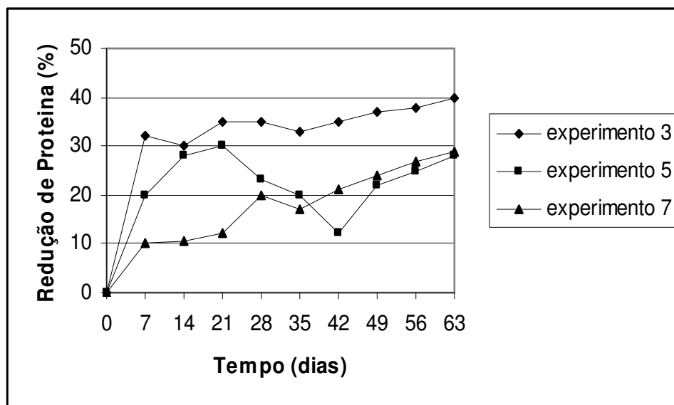
Figura 23 Redução média da concentração de proteína no lodo, nos experimentos 3, 5 e 7 ao longo do tempo de operação
