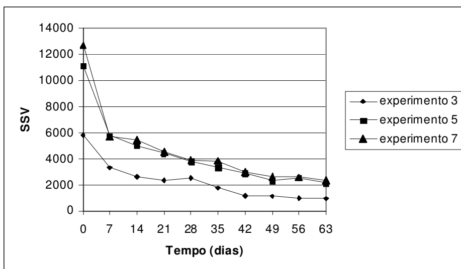
Figura 13 Avaliação média dos SSV nos experimentos 3, 5 e 7 com tempo de operação de 30 dias
