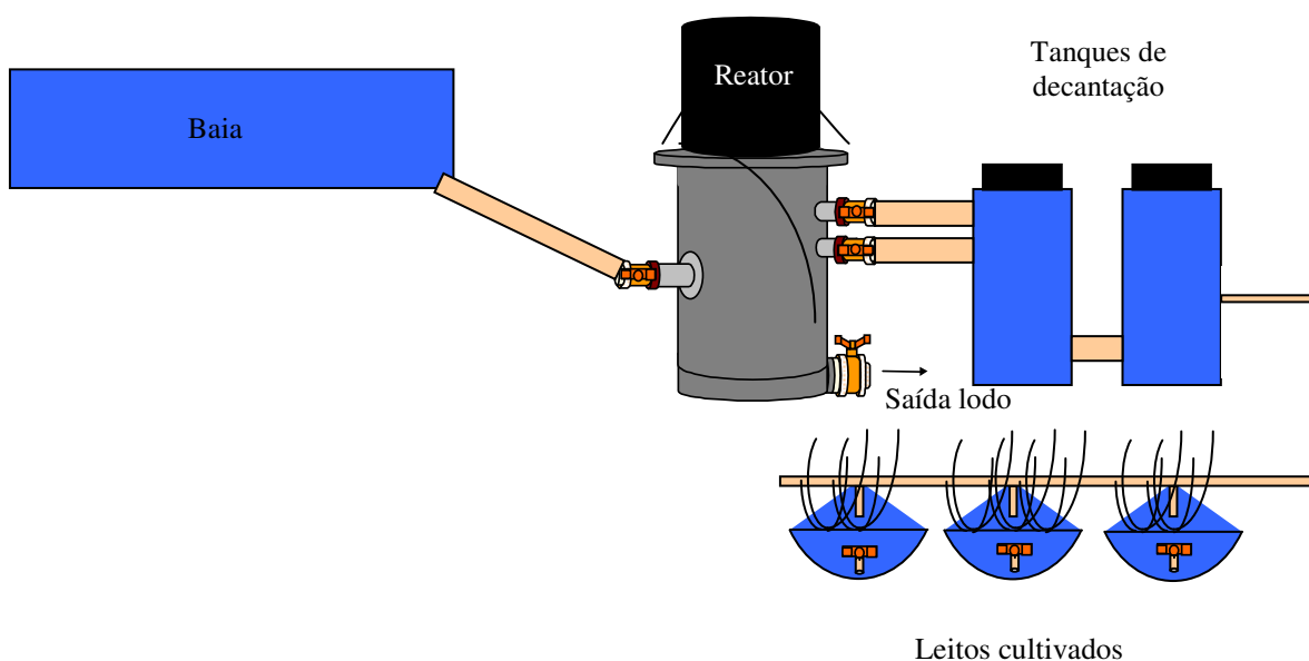
Figura 3.1- Esquema do Sistema Integrado de Tratamento de Dejetos de Suínos
