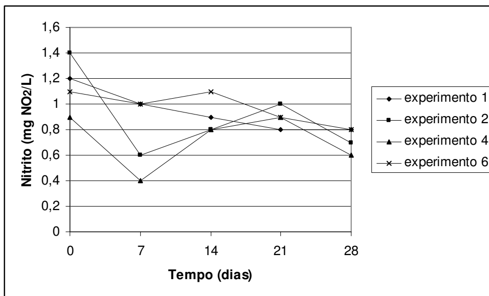
Figura 20 Evolução da concentração de nitrito no sobrenadante, nos experimentos 1, 2, 4 e 6 ao longo do tempo de operação
