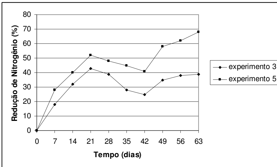
Figura 19 Redução média da concentração de nitrato no sobrenadante, nos experimentos 3, e 5 ao longo do tempo de operação
