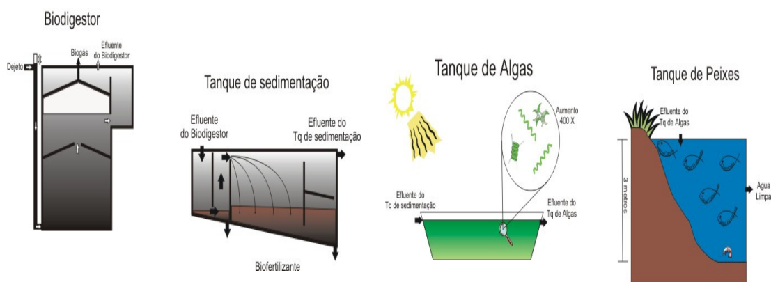
Figura 2.10 - Sistema integrado de tratamento.
