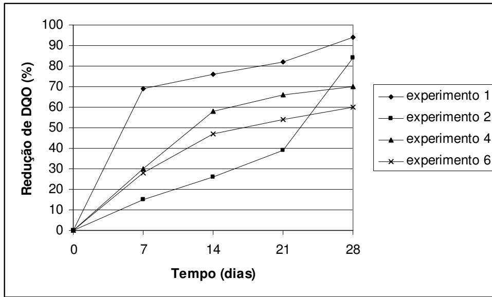
Figura 14 Redução média de DQO total nos experimento 1, 2, 4, e 6 ao longo do tempo de operação
