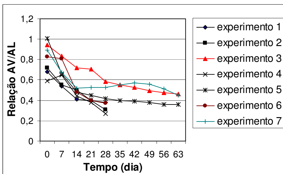
Figura 4.1 – Evolução da relação AV/AL no biodigestor
