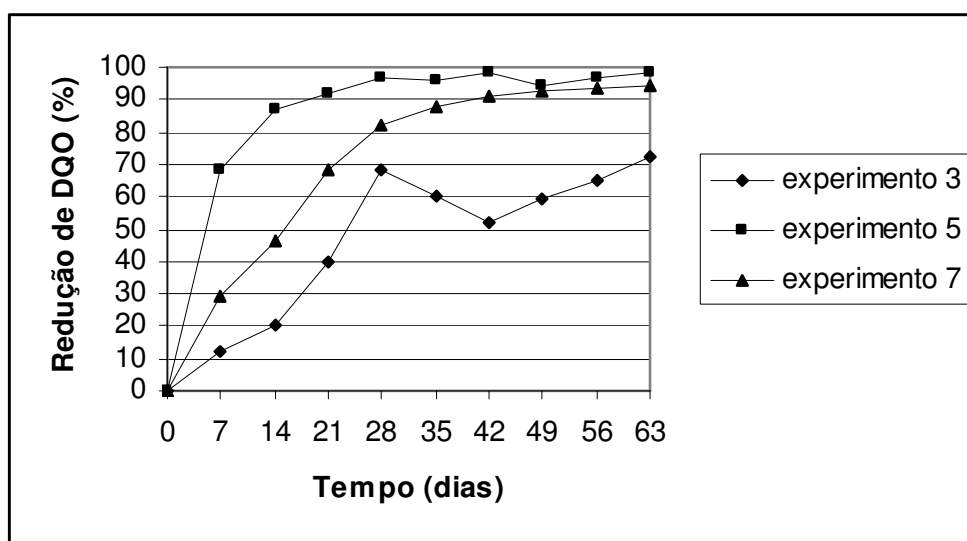
Figura 17 Redução média de DQO solúvel nos experimento 3, 5 e 7 ao longo do tempo de operação
