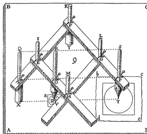
Pantógrafo 6
